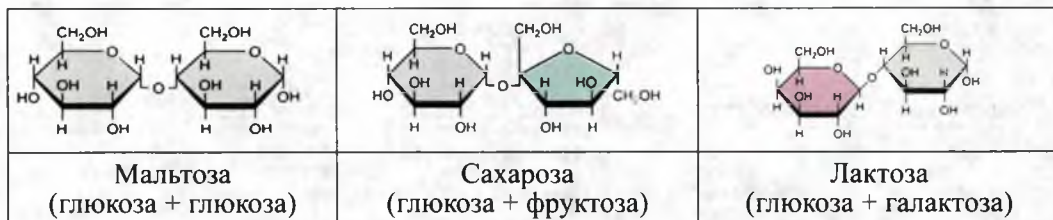
Рис.6. Дисахариды.
