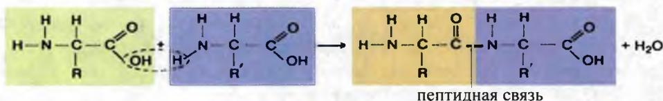
Рис.8. Взаимодействие аминокислот
