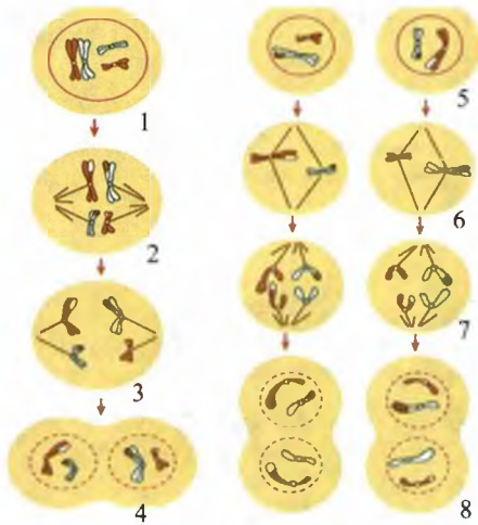
Рис.32. Мейоз.
