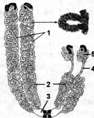
Рис.29. Строение хромосомы.
