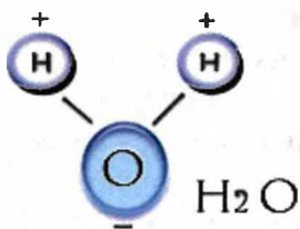
Рис.3. Молекула воды
