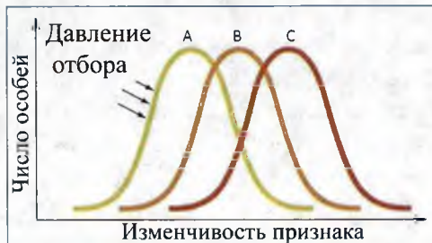
Рис.94. Движущий отбор.
