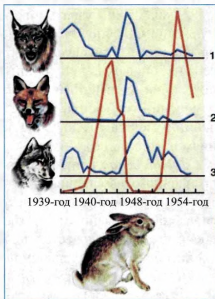
Рис.80. Рост популяций.
