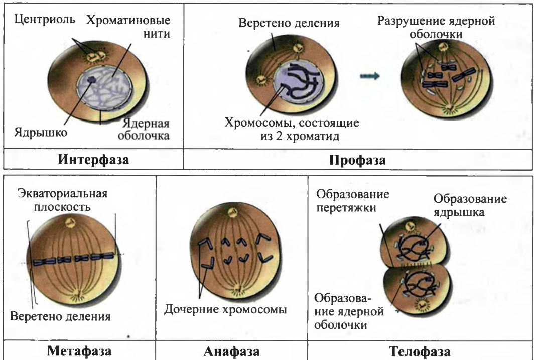
Рис.30. Этапы митоза.
