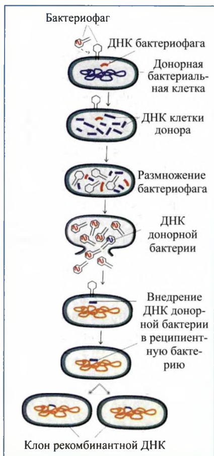
Рис.68. Процесс трансдукции.
