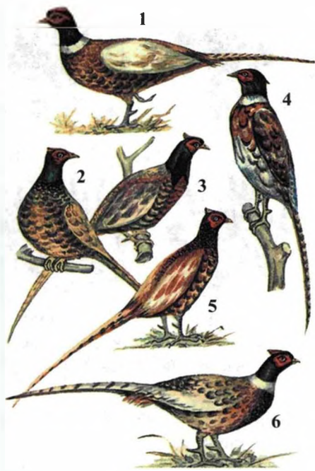
Рис.108. Подвид фазанов.
