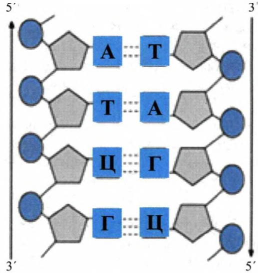
Рис.16. ДНК.
