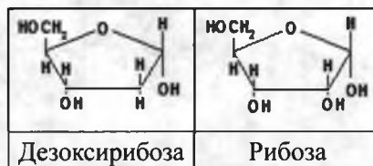
Рис.11. Пентозы.
