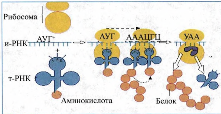
Рис.27. Процесс трансляции.
