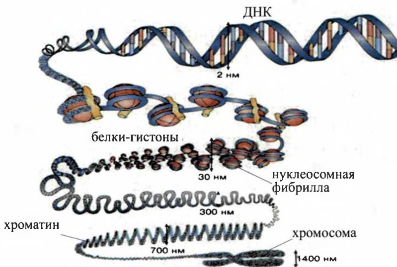
Рис.28. Структура хромосомы.
