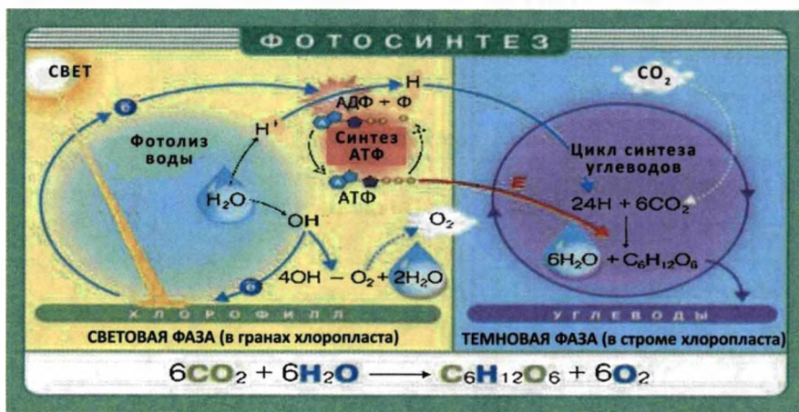
Рис.23. Процесс фотосинтеза.
