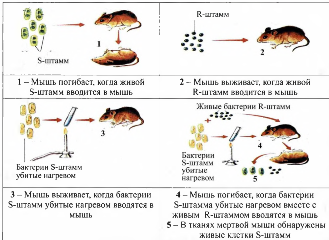
Рис.66. Опыт Гриффита.
