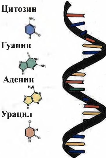
Рис.17. Строение РНК.
