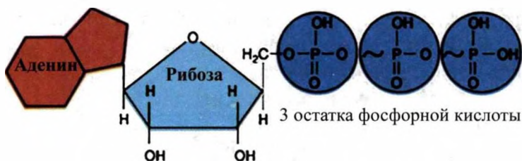
Рис.14. Строение АТФ.
