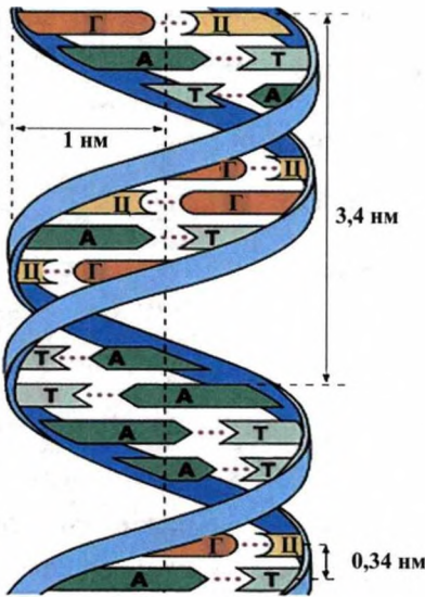
Рис.15. Строение ДНК
