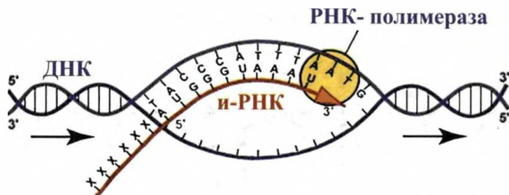
Рис.26. Транскрипция.
